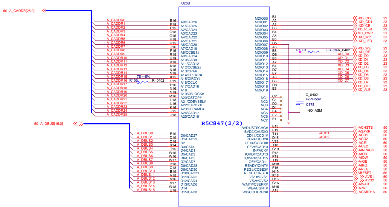
R5C847-CSP208Q 208p_bga_16x16
